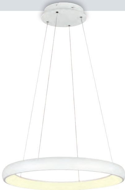
TRIO LED-Pendelleuchte weiß-matt IP20 inkl. DIP-SWITCH Dimmer Helligkeit in 3 Stufen mit herkömmlichen Schalter einstellbar ØxH: 46,5x150cm inkl. SMD-LED-29W CCT 2.300/3.000/4.000K 3.300lm 33226770 126,00 €
